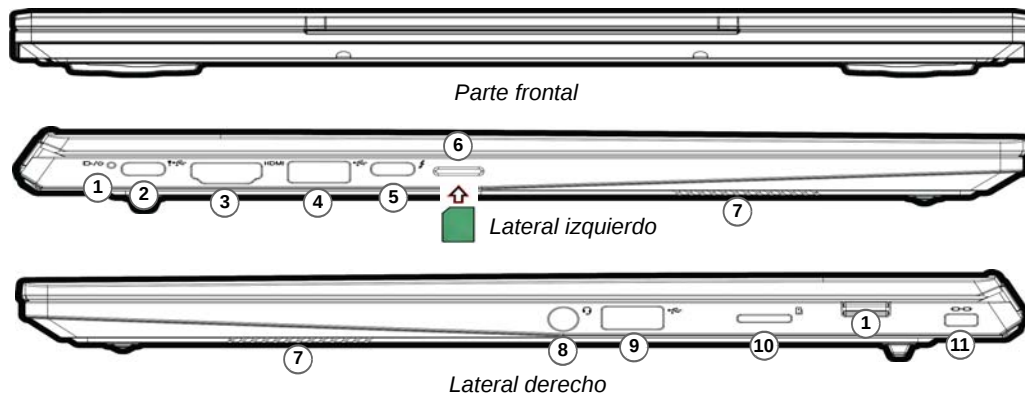
Figura 9 - Vistas frontal, izquierda y derecha (Modelo B)
