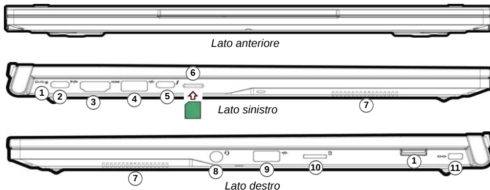
Figura 9 - Vista anteriore, sinistra e destra (Modello B)
