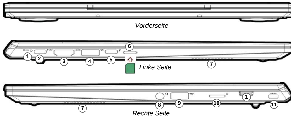
Abb. 8 - Ansicht von vorne, links und rechts (Modell A)
