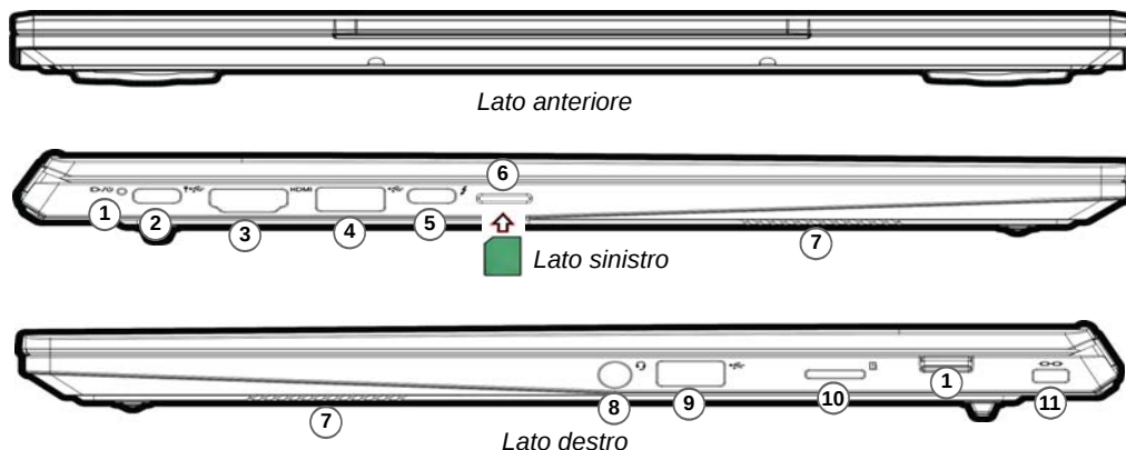
Figura 8 - Vista anteriore, sinistra e destra (Modello A)
