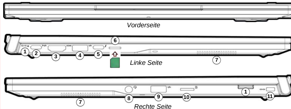
Abb. 9 - Ansicht von vorne, links und rechts (Modell B)
