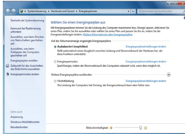
Abb. 31 - Energieoptionen
