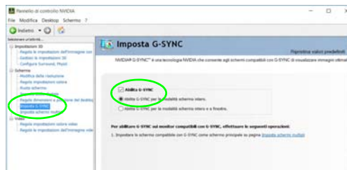
Figura 26 Imposta G-SYNC
