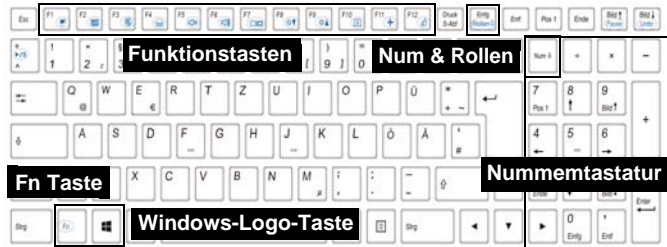
Abb. 6 - Tastatur
