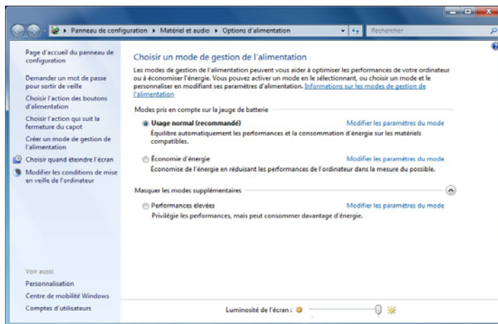
Figure 31 - Options d'alimentation
