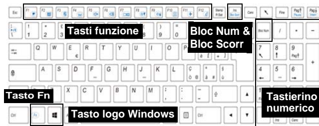
Figura 6 - Tastiera
