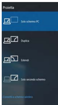
Figura 27 Proietta
