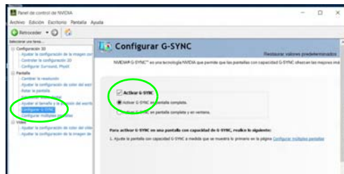
Figura 26 Configurar G-SYNC
