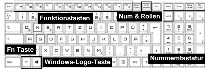
Abb. 5 - Tastatur
