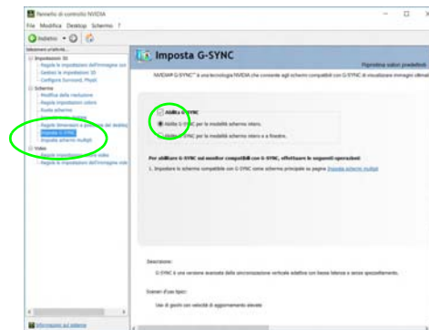
Figura 26 - Imposta G-SYNC
