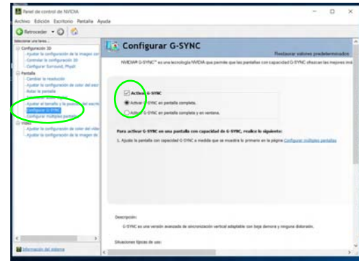
Figura 26 - Configurar G-SYNC
