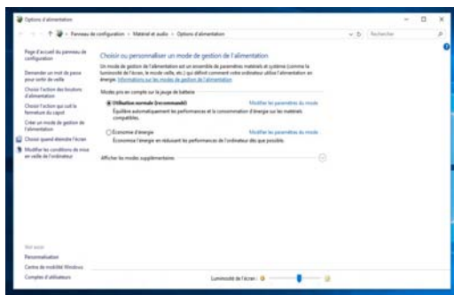
Figure 27 - Options d'alimentation
