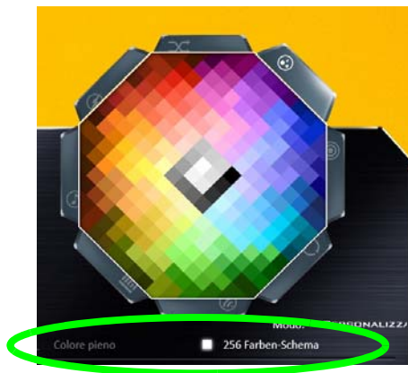
Figura 21 - Campione colore
