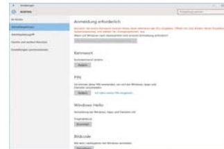
Abb. 31 Konten - Anmeldeoptionen
