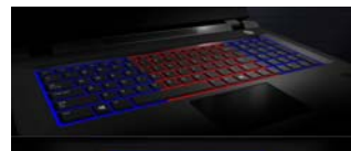
Figura 22 Anteprima
