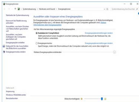
Abb. 27 - Energieoptionen
