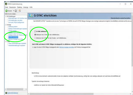
Abb. 26 - G-SYNC einrichten
